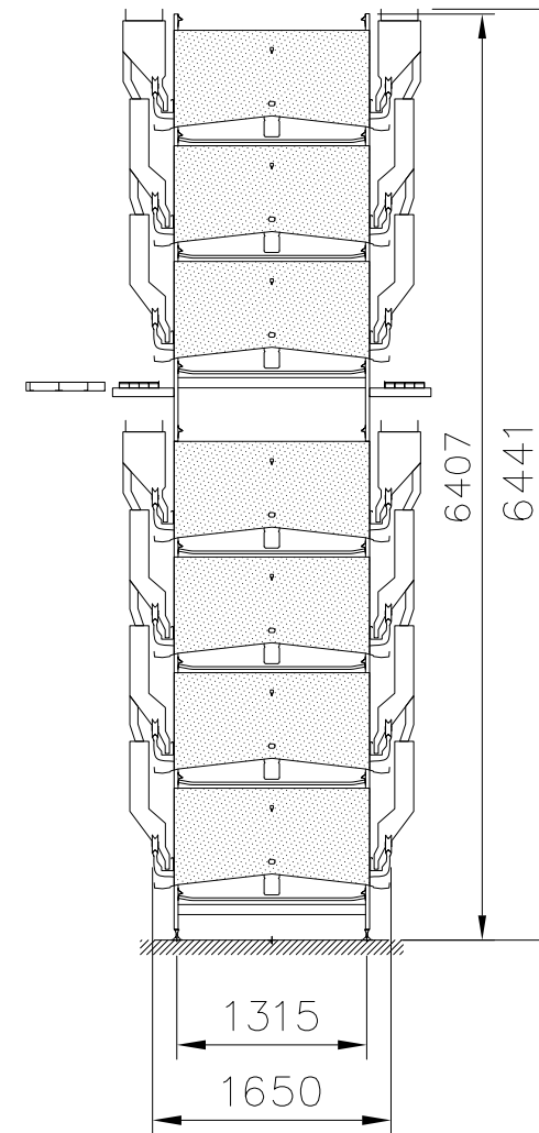
Modulo Famiglia MF135 - 4+3 tiers
