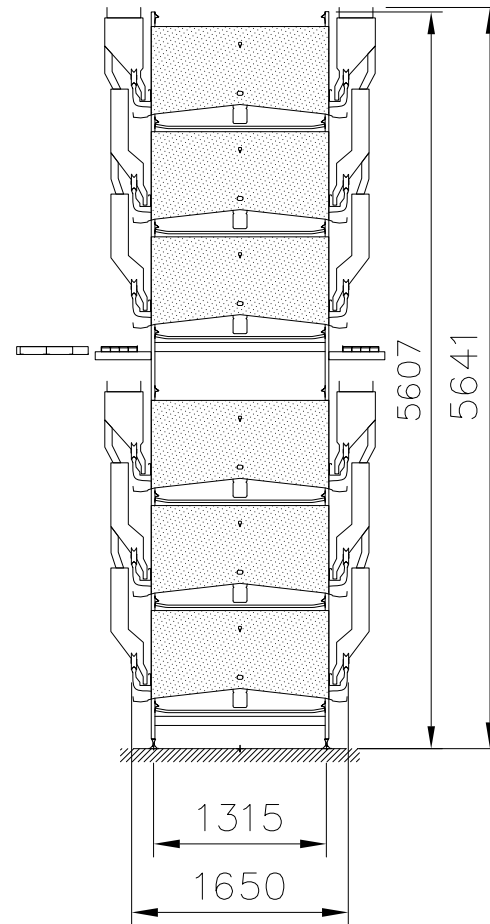
Modulo Famiglia MF135 - 3+3 tiers
