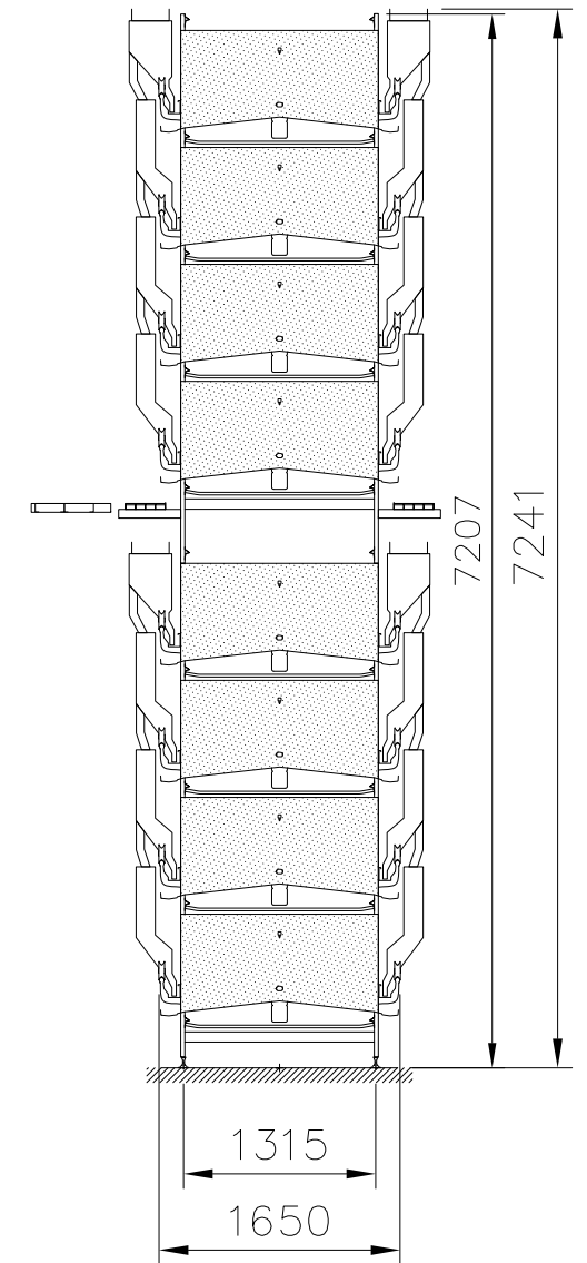
Modulo Famiglia MF135 - 4+3 tiers
