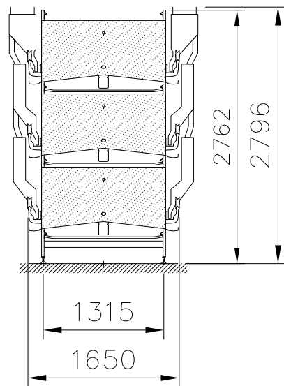
Modulo Famiglia MF135 - 3 tiers
