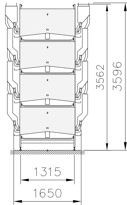
Modulo Famiglia MF135 - 4 tiers
